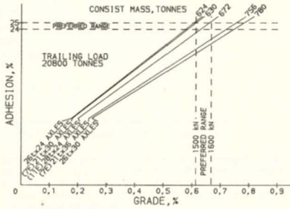
Fig. 1 Graphical Optimisation
